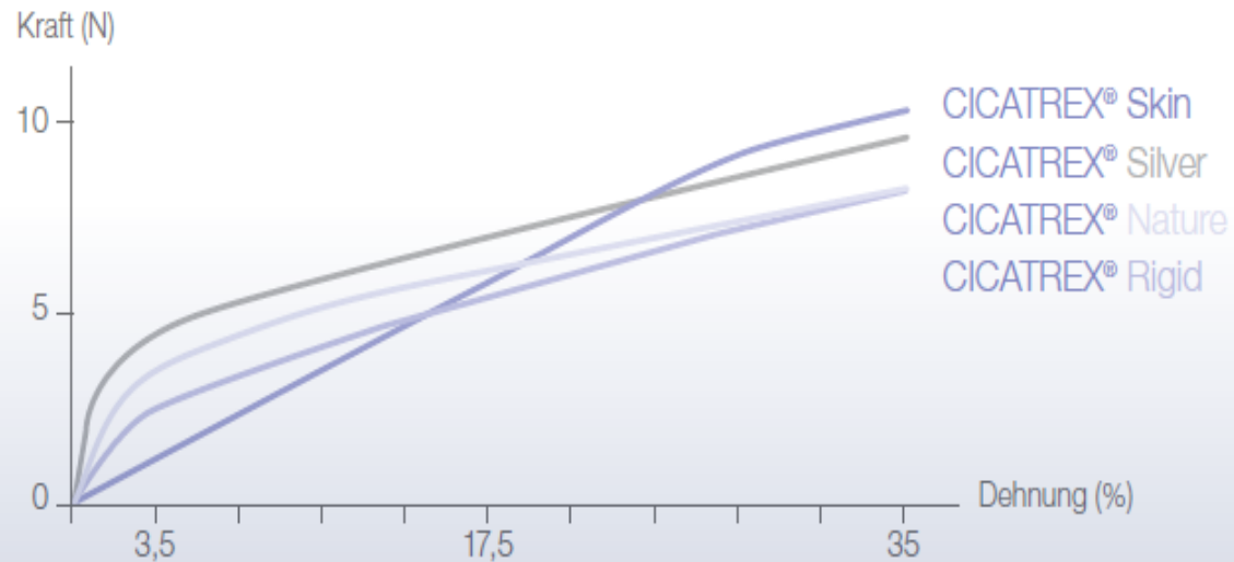
Druck-Dehnungskurve
